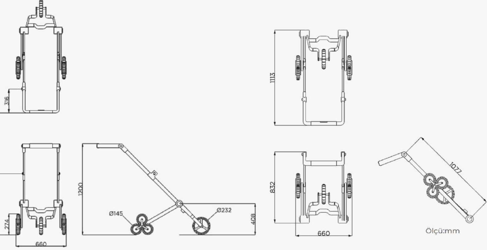
Teknik Çizim Kargo taşıma strüktürü
