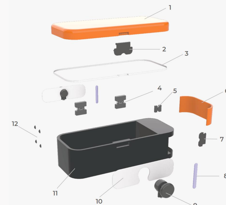
Teknik Çizim Modül 2
