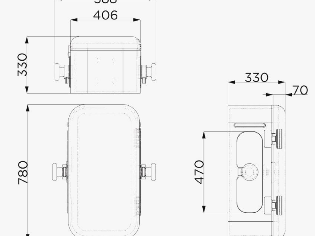
Teknik Çizim Modül 2
